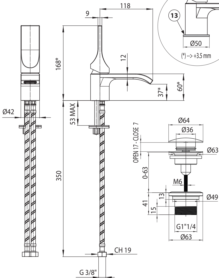
E89600 - Basin mixer
