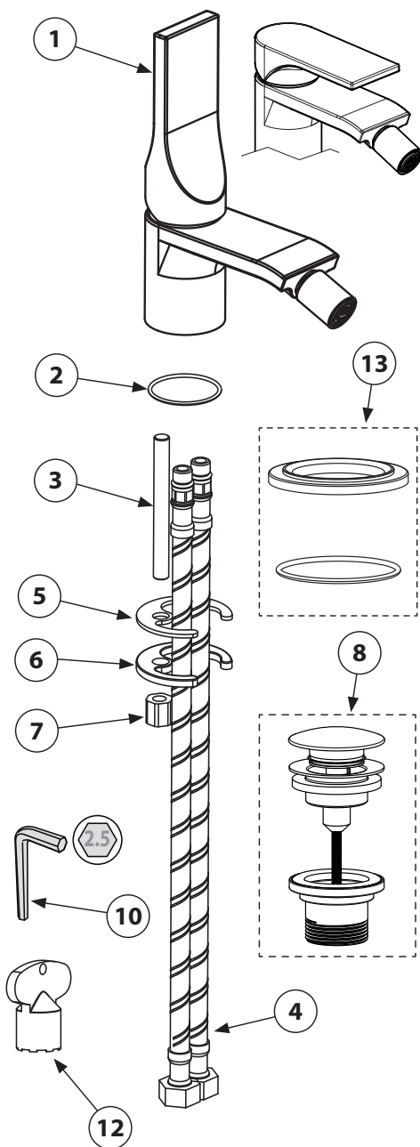
E89601 - E89606 Bidet mixer
