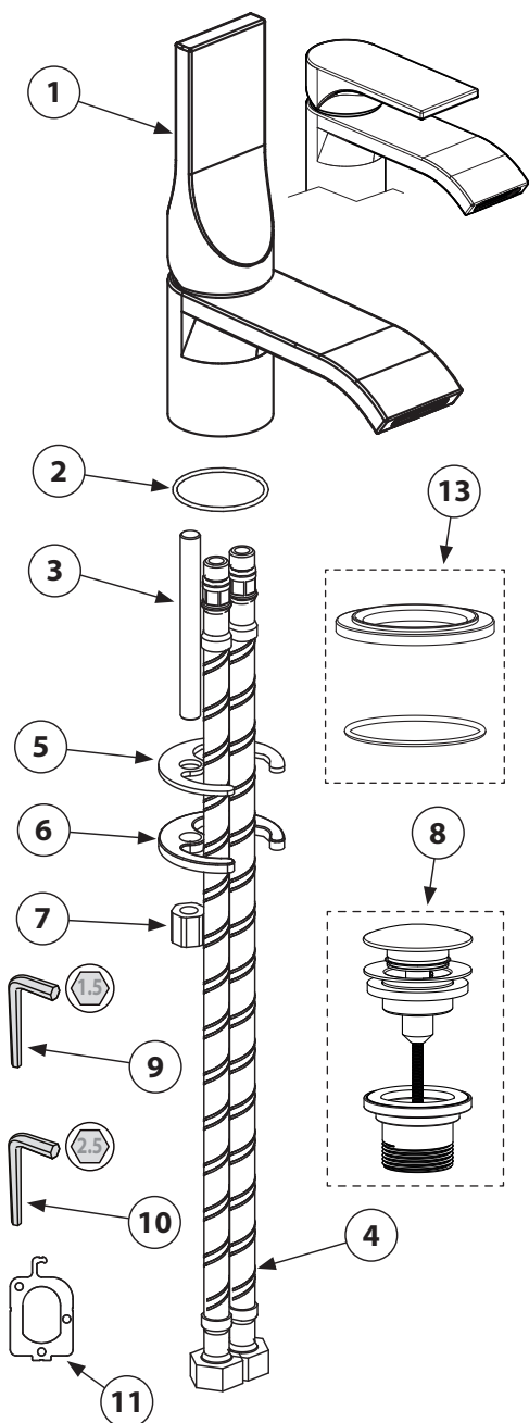
E89600 - E89605 Basin mixer
