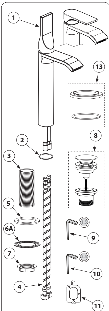
E89602 - E89607 -- High basin mixer E89603 - E89608 -- Middle size basin mixer
