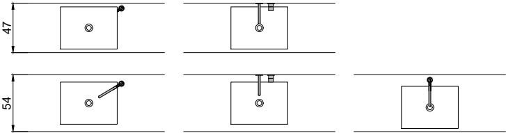
schema d' installazione lavabi e rubinetteria / sinks and taps installation layout
