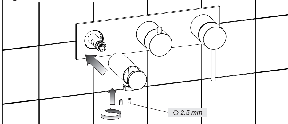
Fig. 15 - Art. 54038-54040
