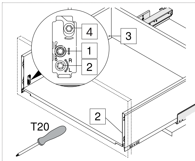
10_ Регулировка ящика.
