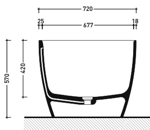
sezione laterale / section
