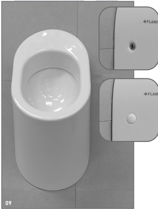
09 Installazione dell'orinatoio: montare il sanitario a parete, dopo aver ben lubrificato la guarnizione in gomma del sifone ed il morsetto. Bloccare il sanitario a parete come in figura. Installation of the urinal: mount the sanitary fixture to the wall after lubricating the rubber washer of the siphon and holdfast. Securely fasten the sanitary fixture to the wall as shown in the figure.
