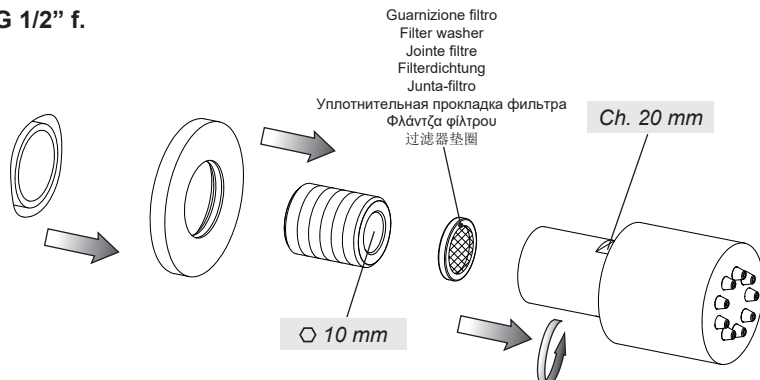
Fig. 6 - G 1/2" m.
