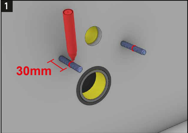
1 Segnare le barre filettate che escono dalla cassetta di scarico a 30mm di distanza dal muro.
